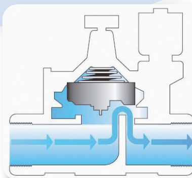
Κλασική σχεδίαση υπο γωνία
