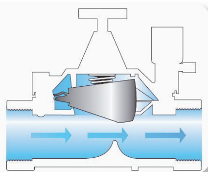
Η σειρά Ultra flow ευθείας ροής
